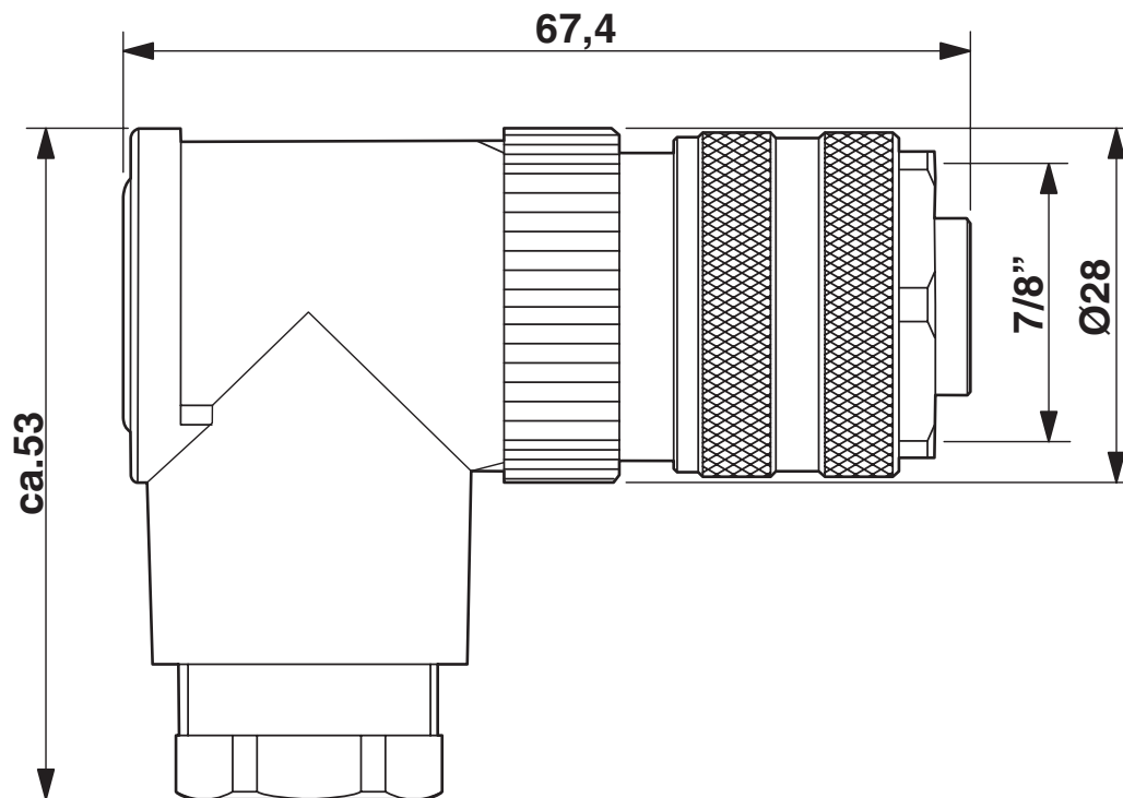
Disegno quotato
