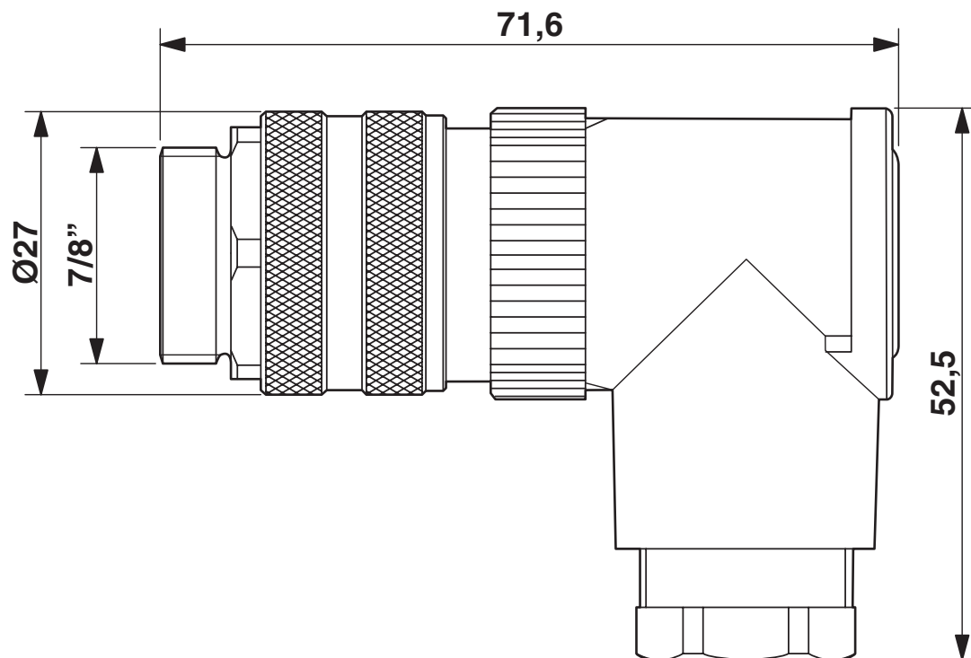
Disegno quotato
