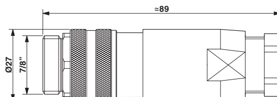
Disegno quotato
