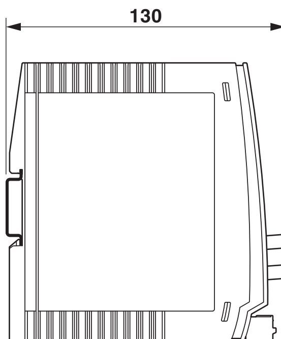
Disegno quotato
