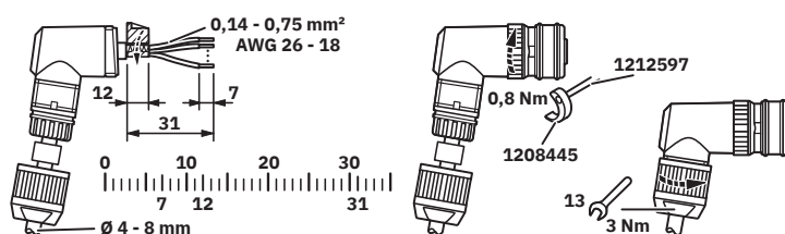
Disegno funzionamento
