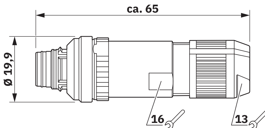
Disegno quotato
