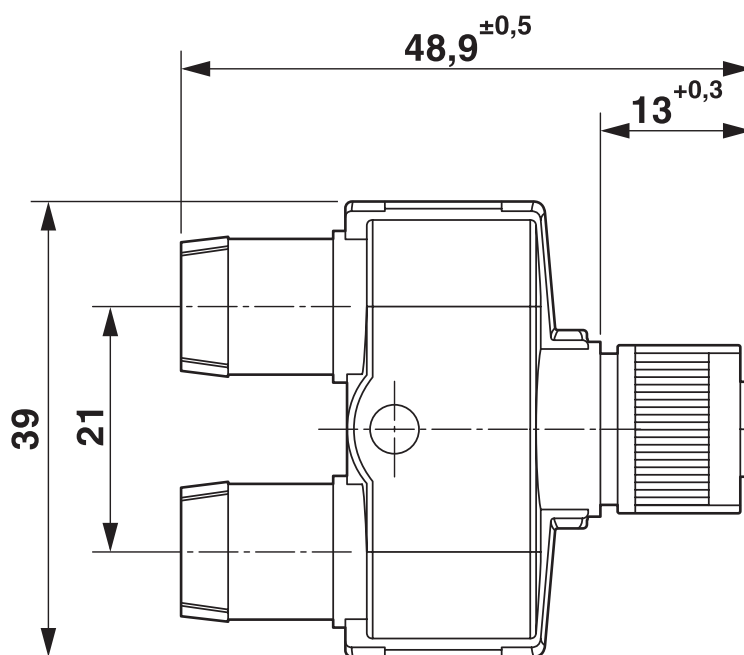
Disegno quotato
