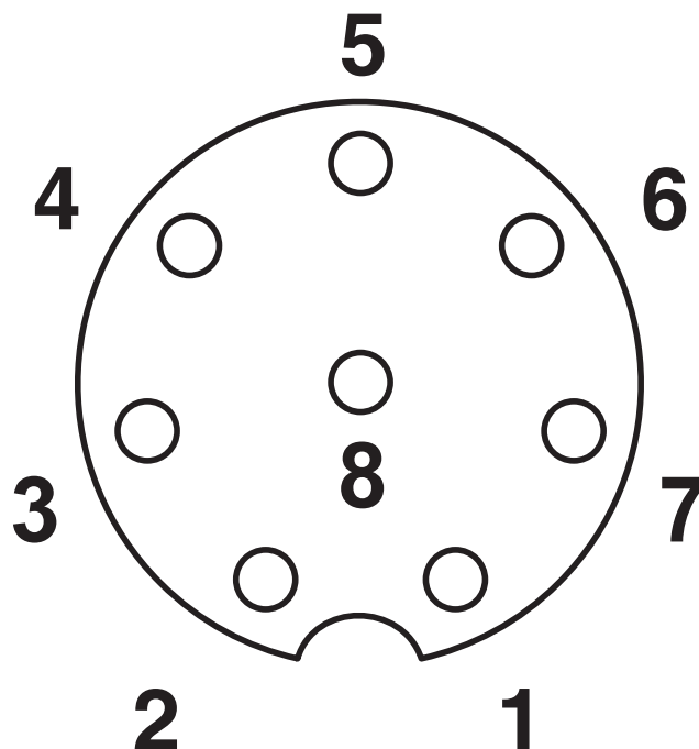
Pinning connettore femmina M12, 6 poli, vista lato femmina
