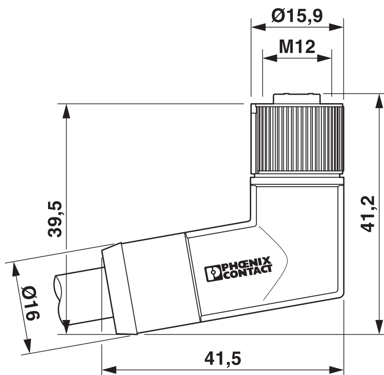
Disegno quotato
