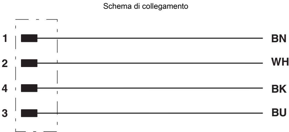
Equipaggiamento dei contatti del connettore M12
