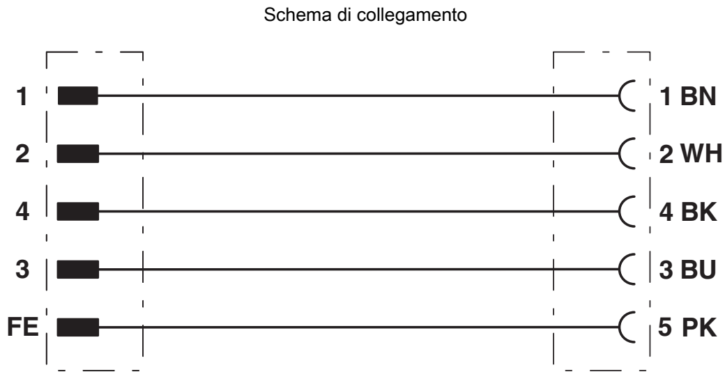
Equipaggiamento dei contatti del connettore maschio/connettore femmina M12
