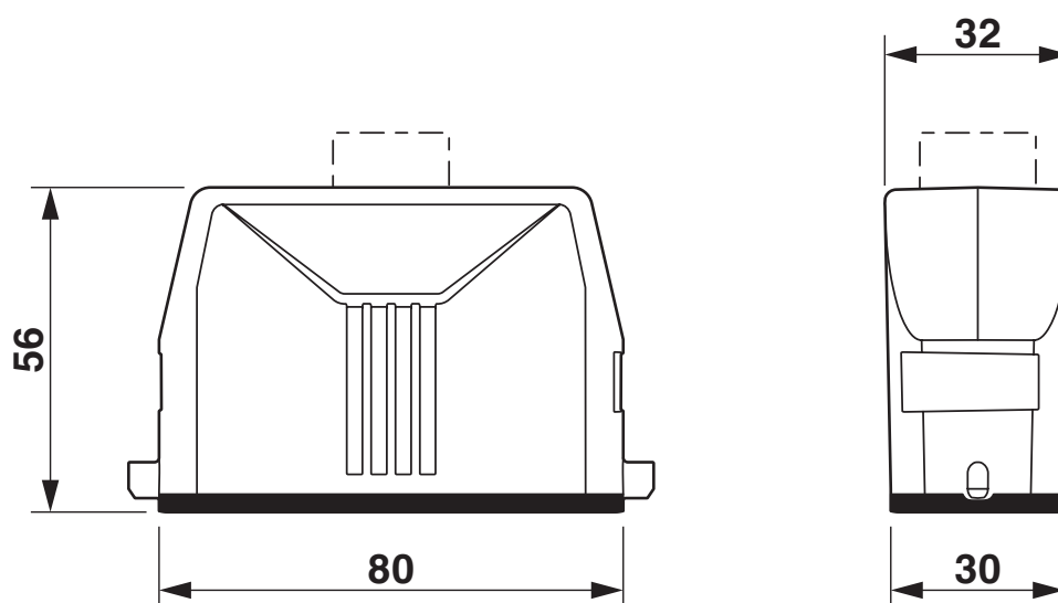
Disegno quotato
