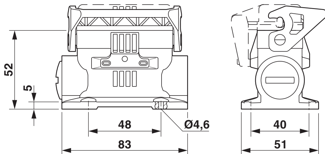
Disegno quotato
