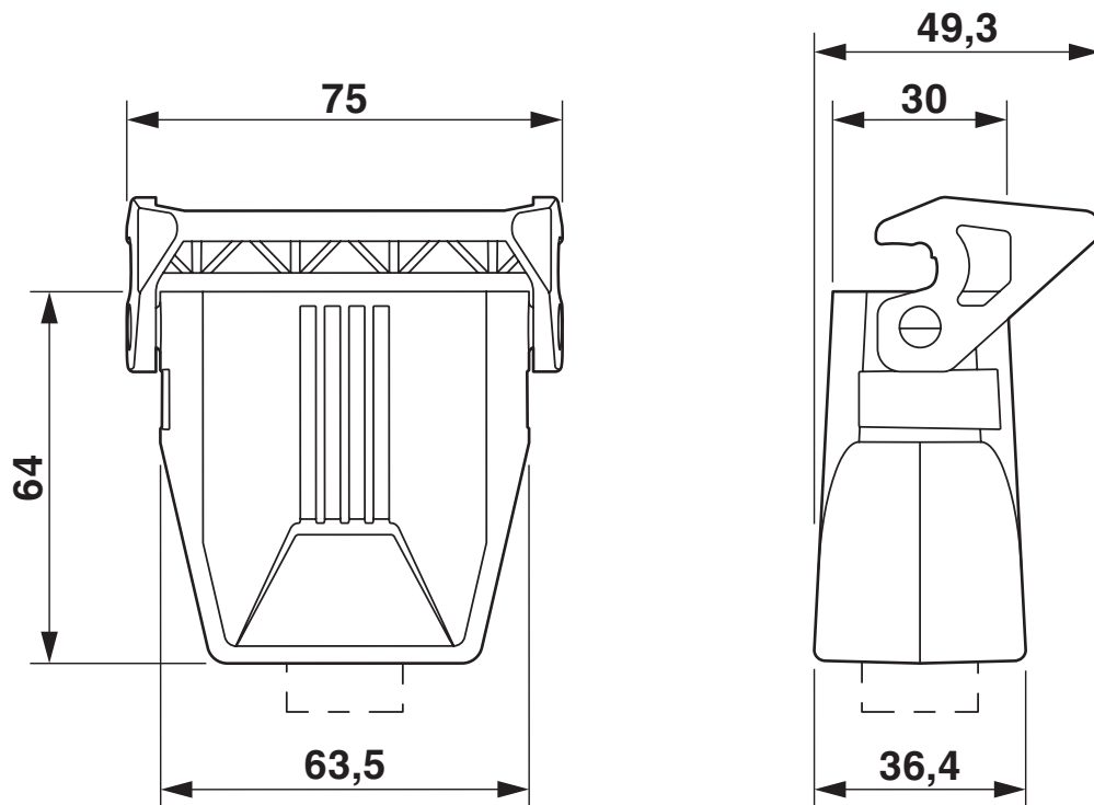
Disegno quotato
