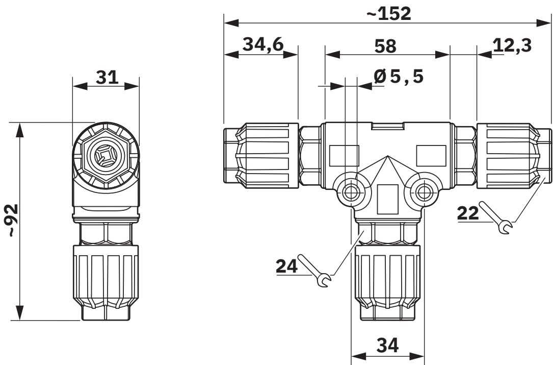
Disegno quotato
