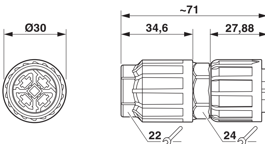
Disegno quotato
