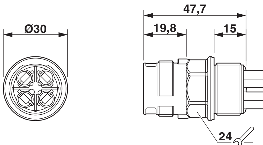
Disegno quotato
