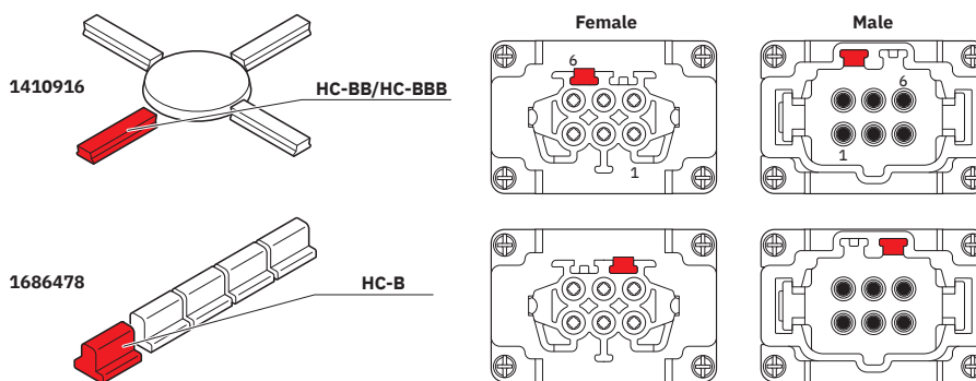
Disegno schema
