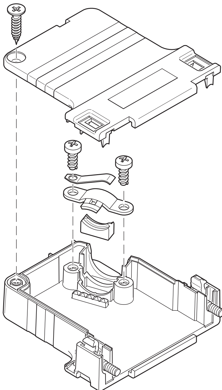
Disegno schema
