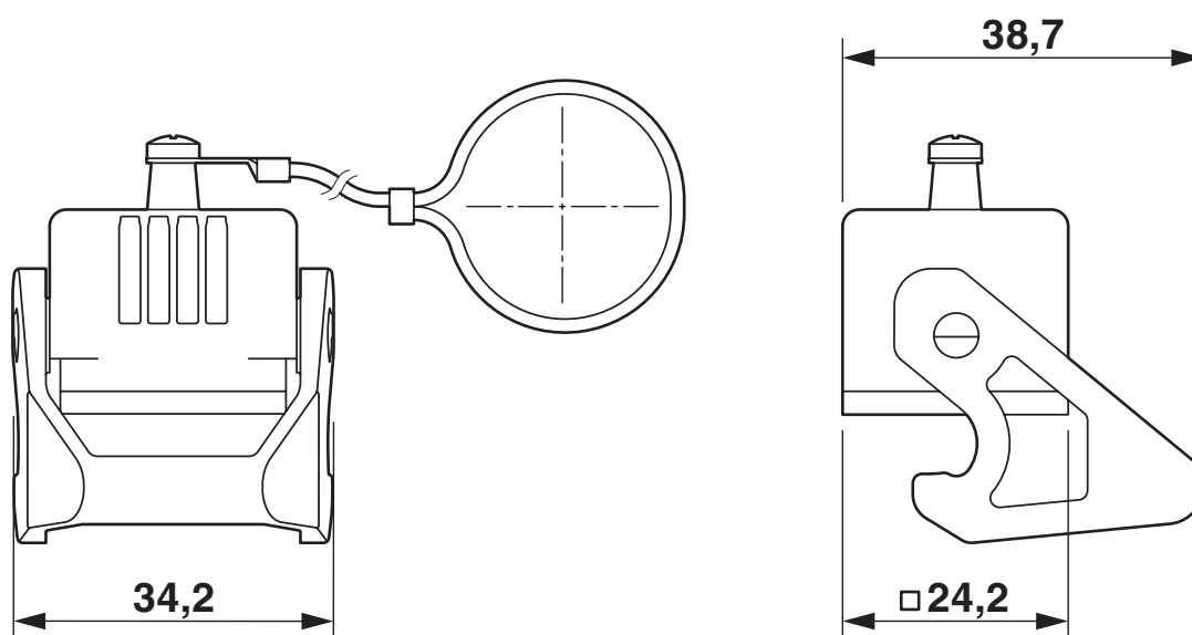
Disegno quotato
