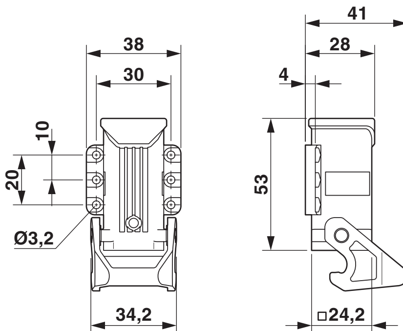
Disegno quotato
