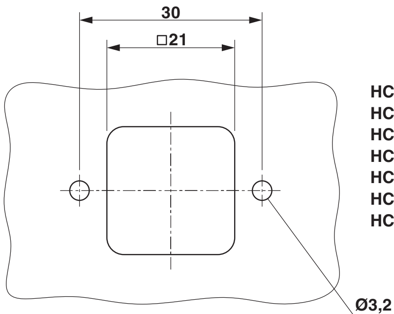
Disegno quotato
