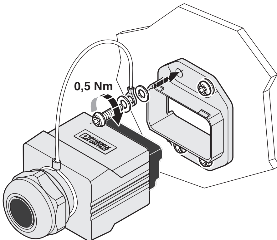
Montaggio del coperchio di protezione
