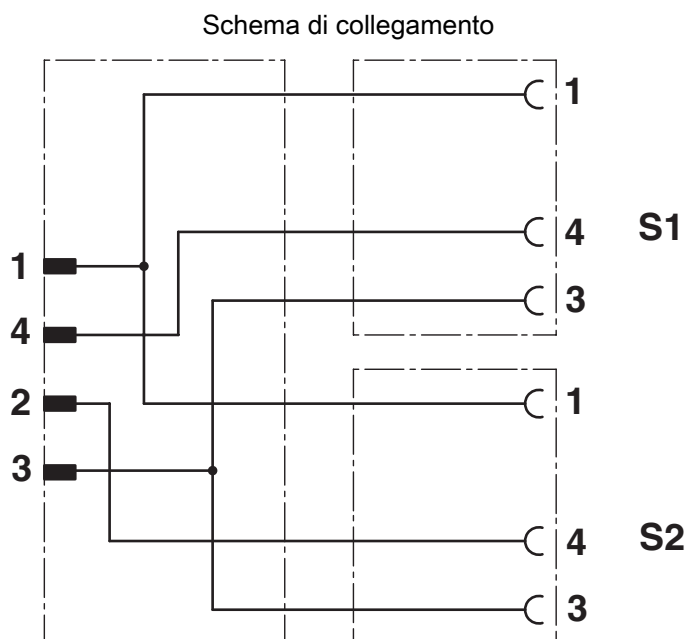
Equipaggiamento contatti connettore maschio M12 e connettore femmina M8
