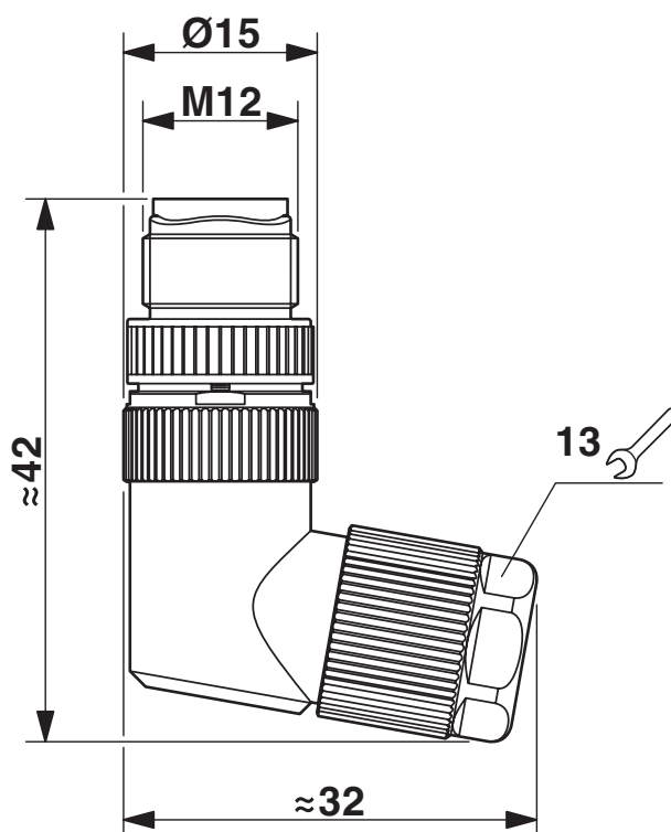
Disegno quotato
