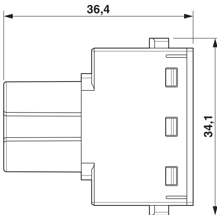
Disegno quotato
