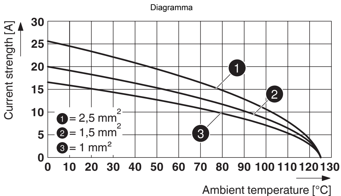
Diagramma di derating (6 moduli in custodia HC-B 24)
