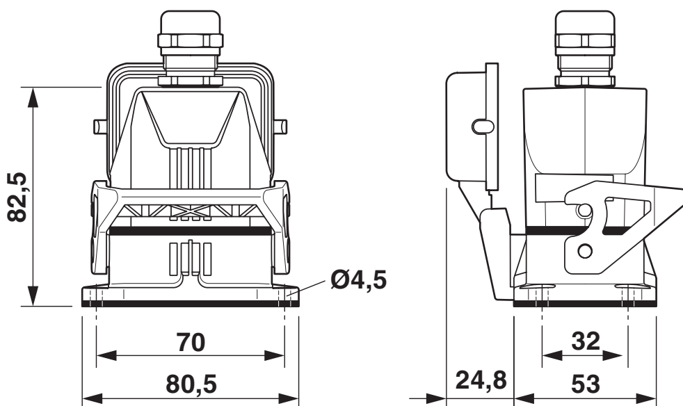
Disegno quotato
