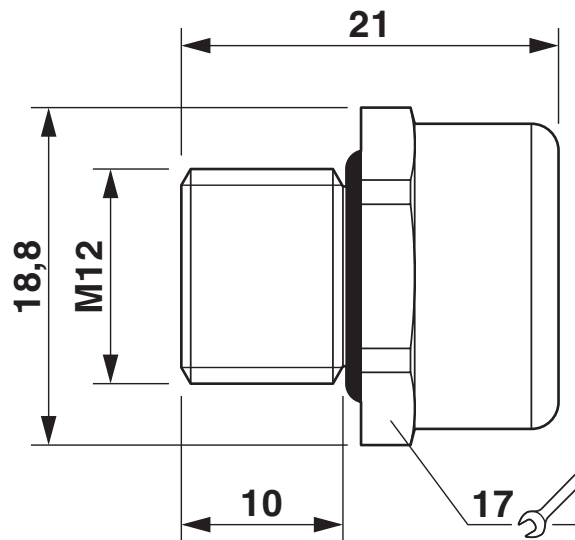
Disegno quotato
