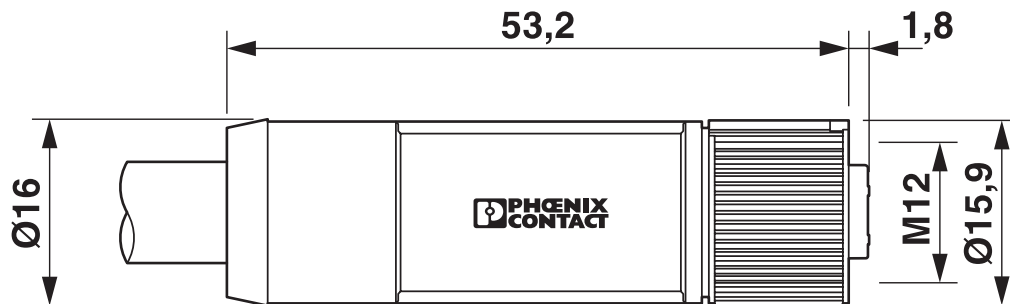
Disegno quotato
