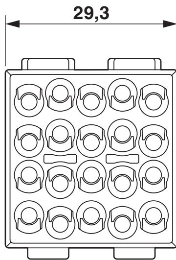
Inserto portacontatti femmina
