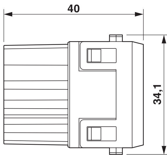
Disegno quotato
