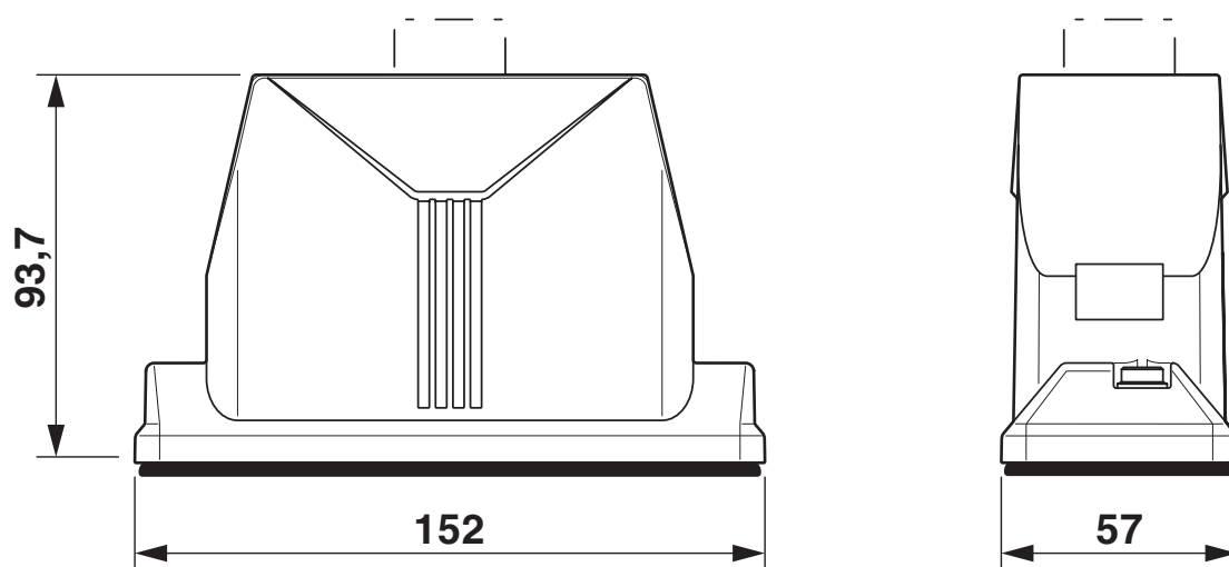
Disegno quotato
