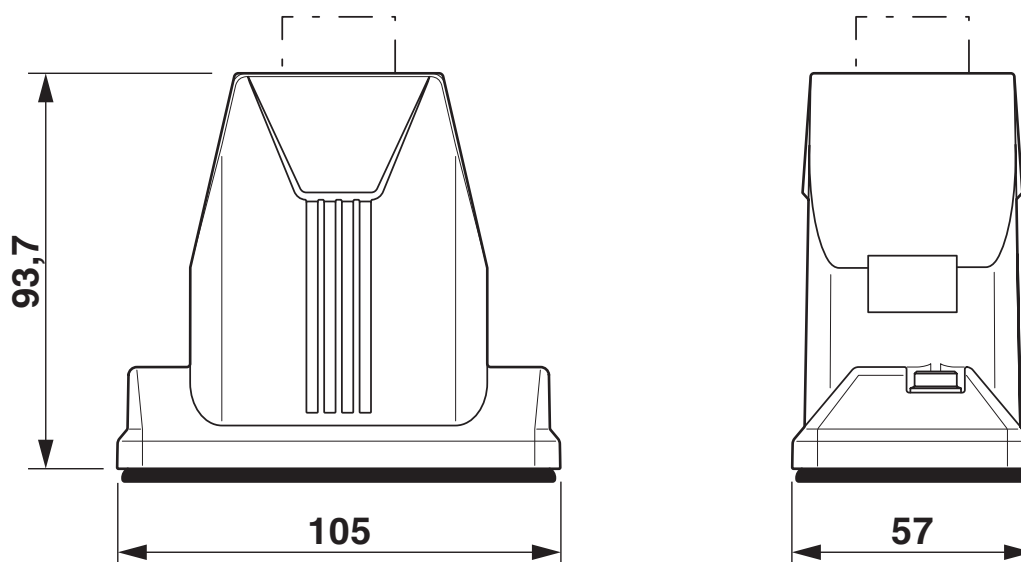
Disegno quotato
