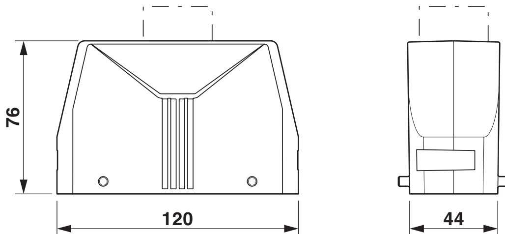
Disegno quotato
