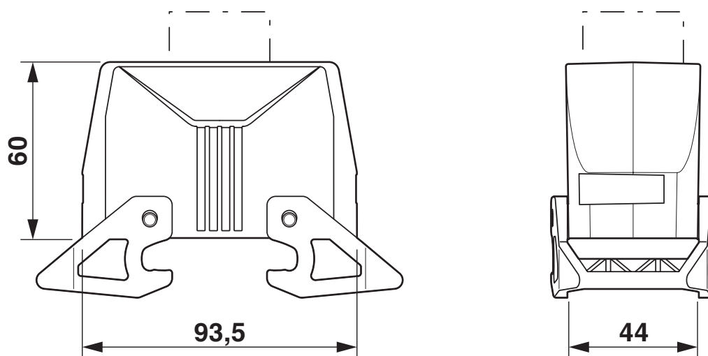
Disegno quotato
