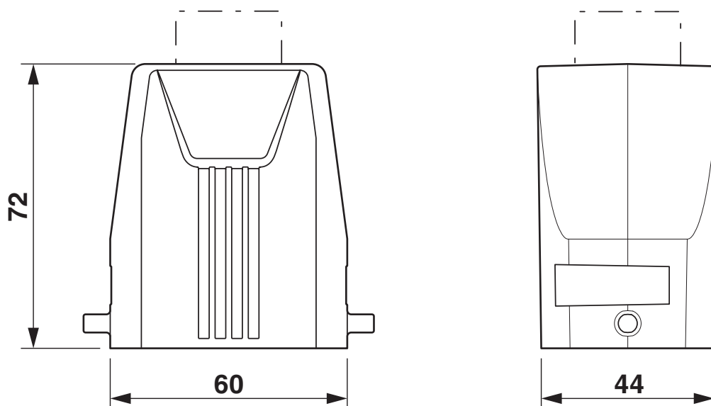
Disegno quotato
