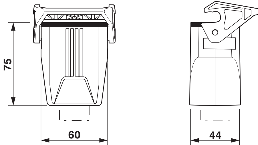
Disegno quotato
