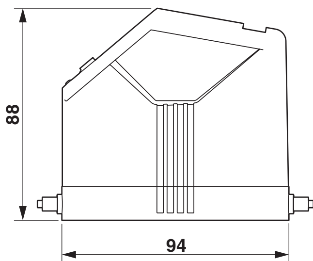
Disegno quotato
