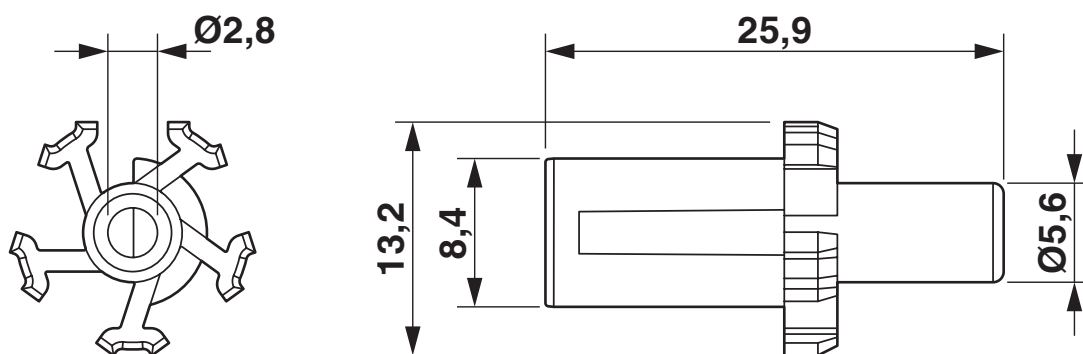
Disegno quotato
