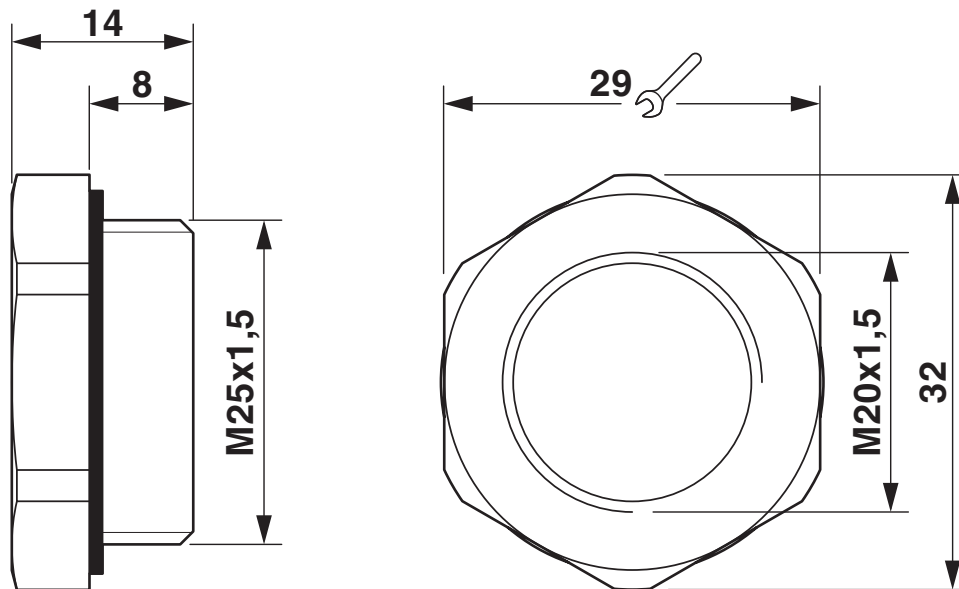
Disegno quotato
