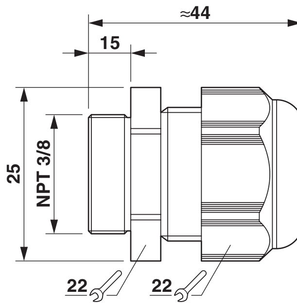
Disegno quotato
