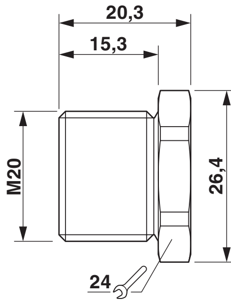
Disegno quotato
