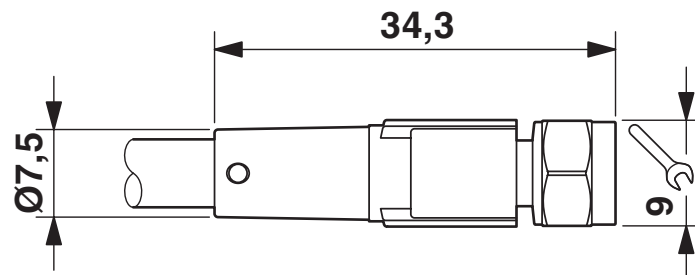
Disegno quotato
