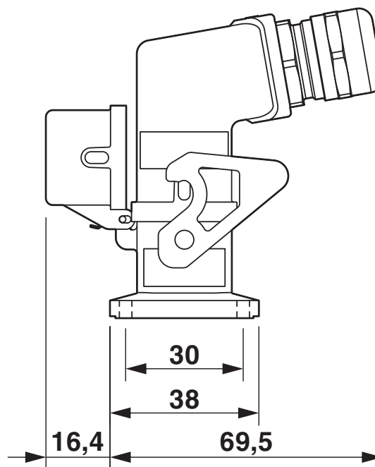
Disegno quotato
