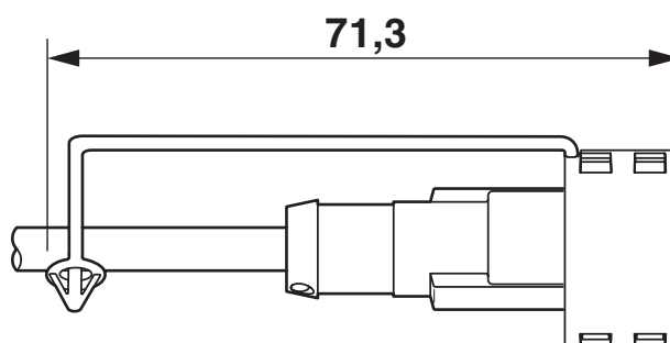
Disegno quotato
