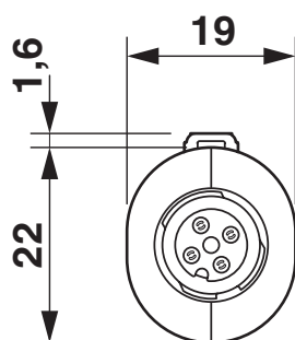
Connettore maschio montato con EXCLIP
