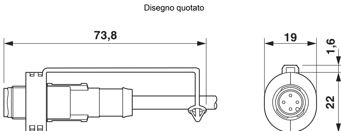
Connettore maschio EXCLIP
