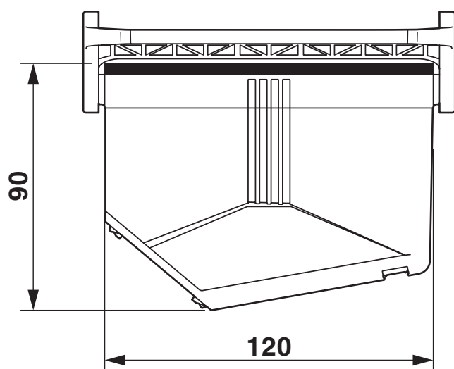
Disegno quotato
