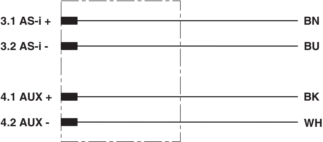
Pinning dei contatti del distributore dell'interfaccia AS
