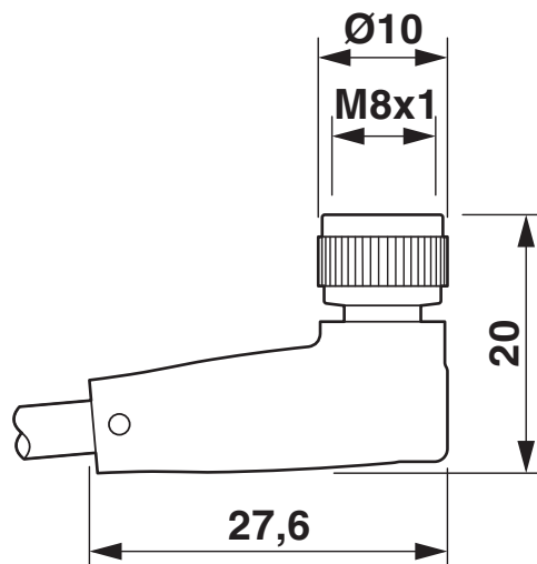
Disegno quotato
