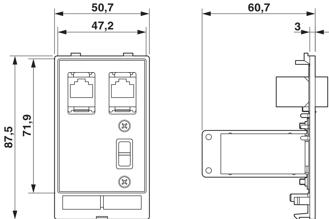
Disegno quotato
