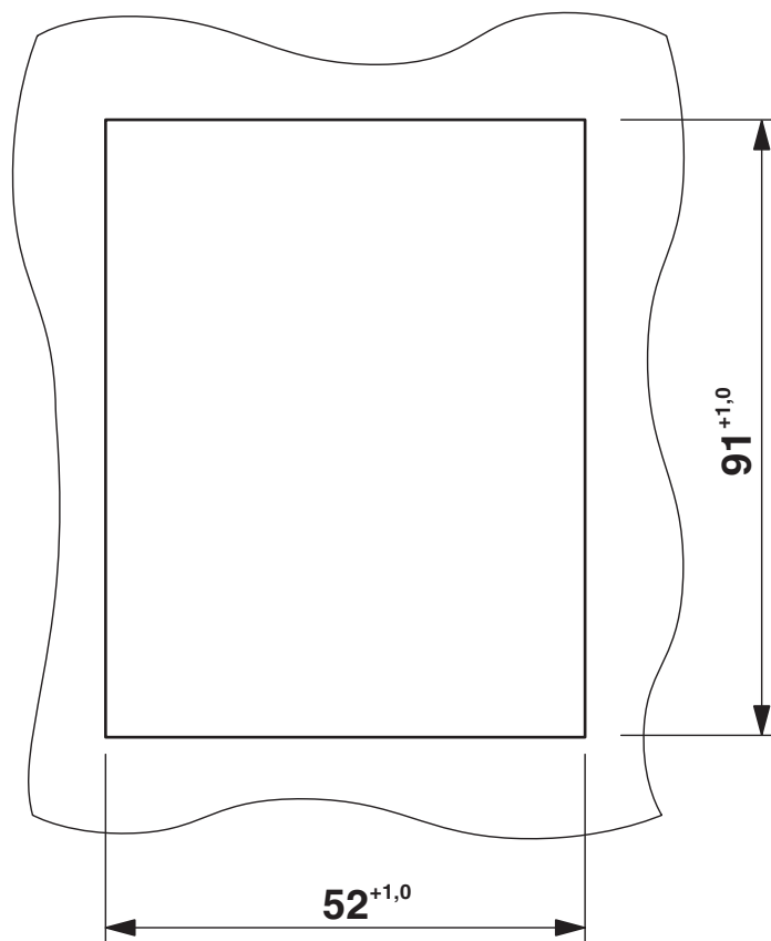
Disegno quotato
